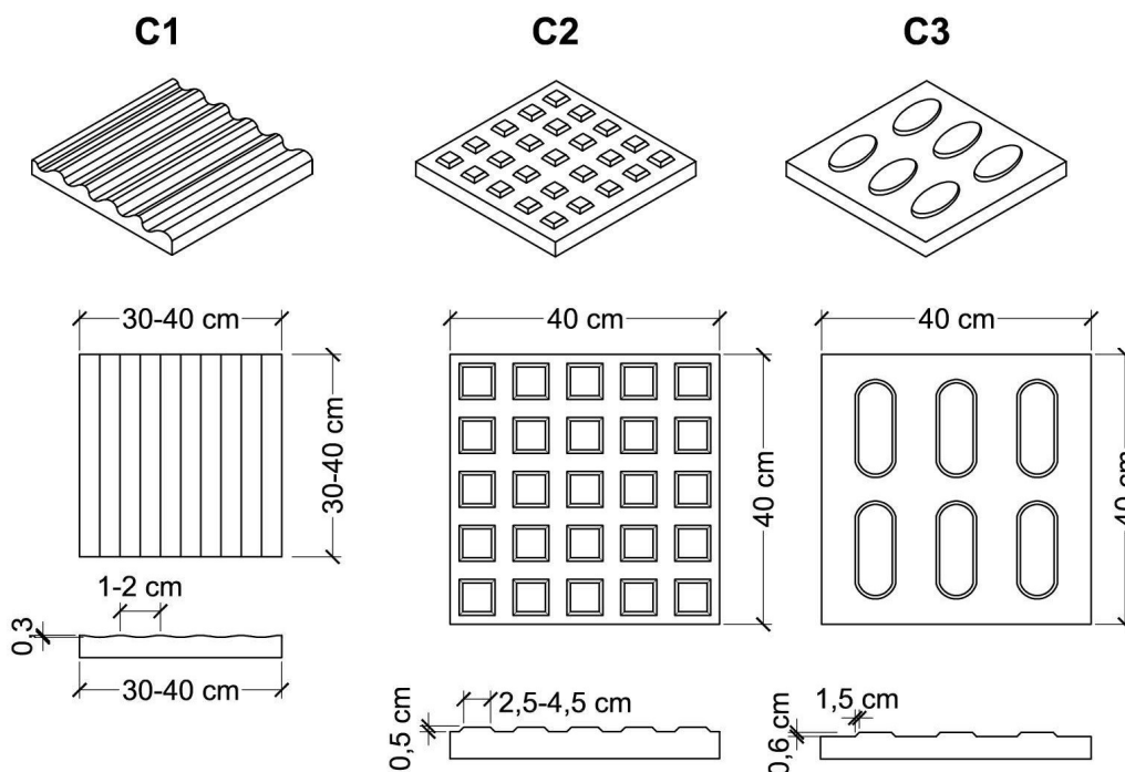
Rys. 16 [25] . Faktury informacyjne - typ C
