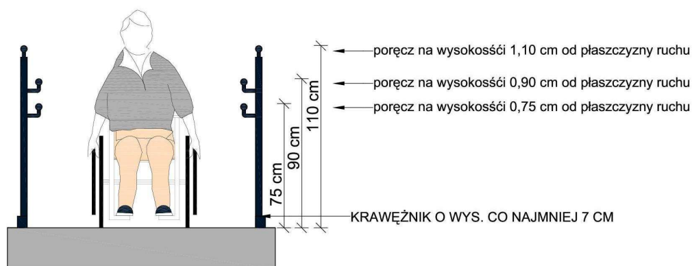
Rys. 32. Zabezpieczenia rampy.
