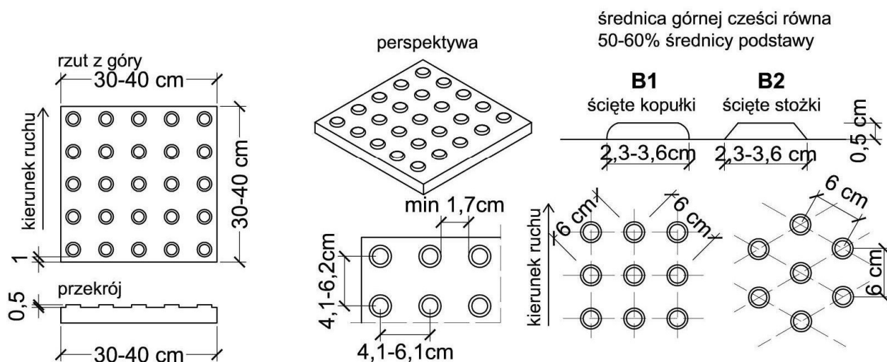
Rys. 15. [24] Faktura bezpieczeństwa, tzw. B1 „ścięte kopułki”, B2 „ścięte stożki”.
