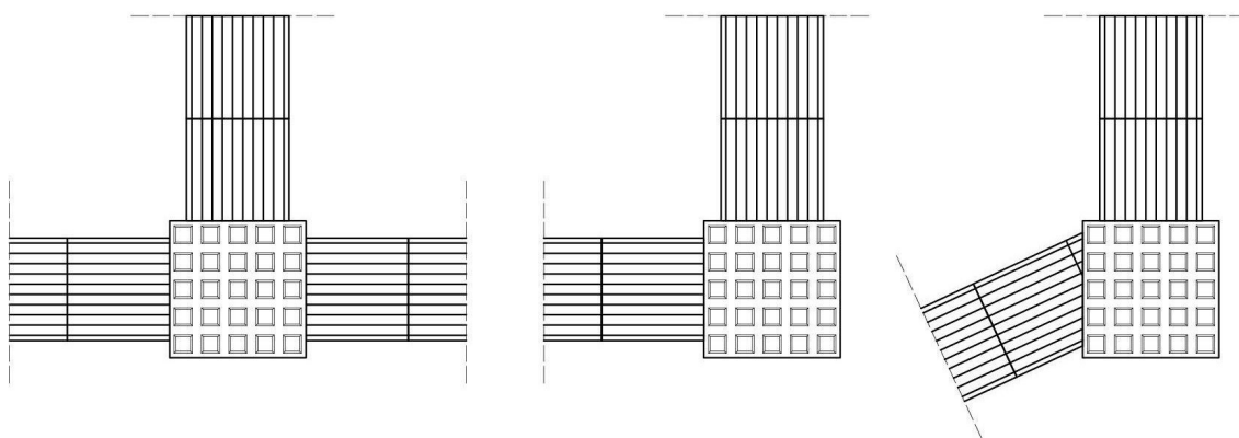
Rys. 19. Przecięcie ścieżek kierunkowych lub zmiana kierunku ścieżki o więcej niż 45 stopni;
