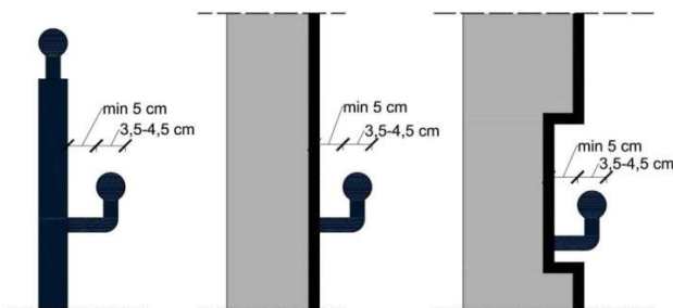
Rys. 33. Poręcz- rozwiązanie poprawne
