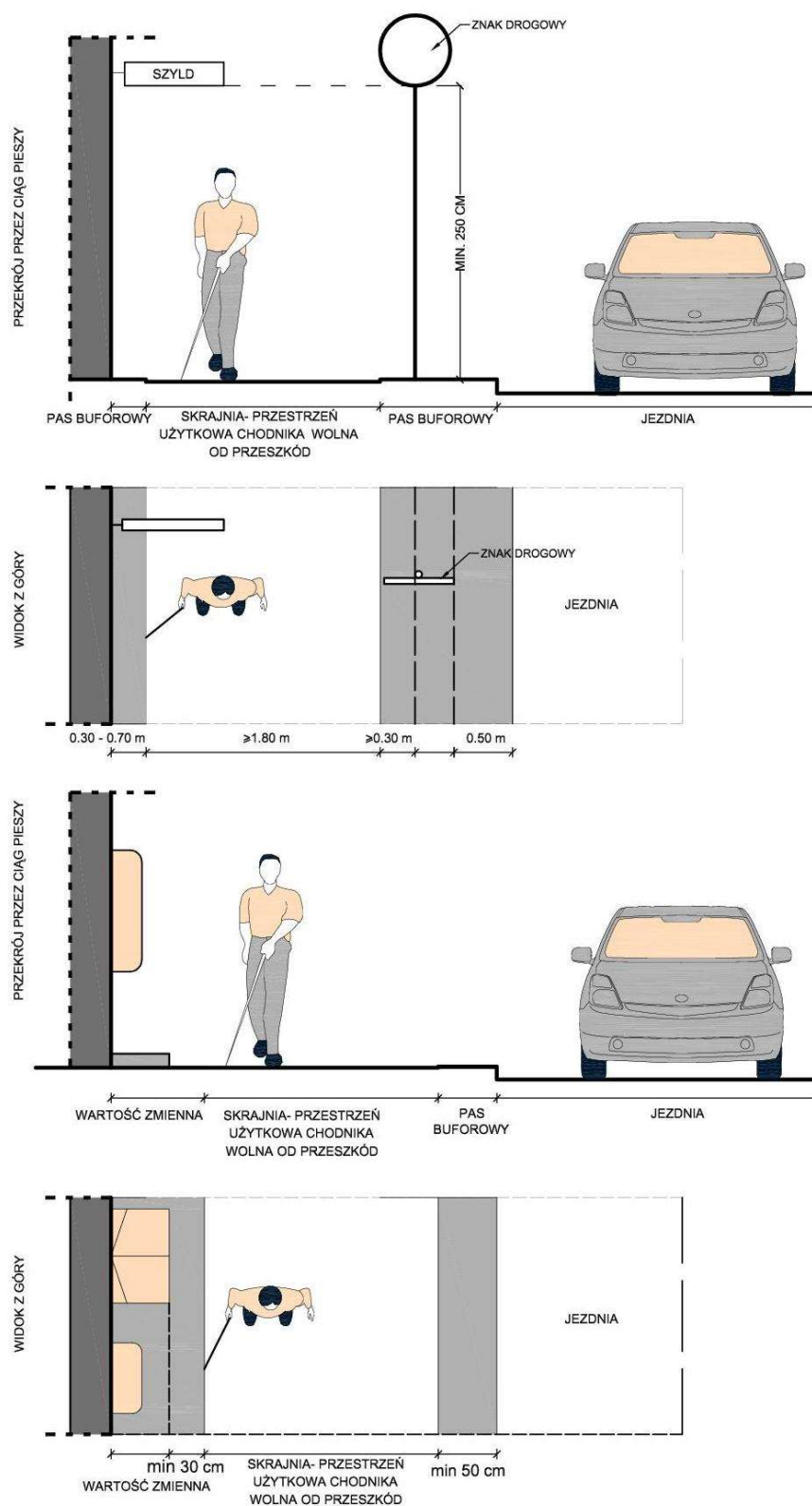
Rys. 5. [21] Sposób zagospodarowania bezpiecznego ciągu pieszego wzdłuż linii zabudowy i przy jezdni.
