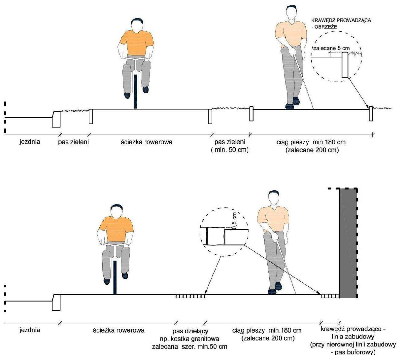
Rys. 7. Zalecana lokalizacja ciągu pieszego i ścieżki rowerowej w pasie drogowym;
