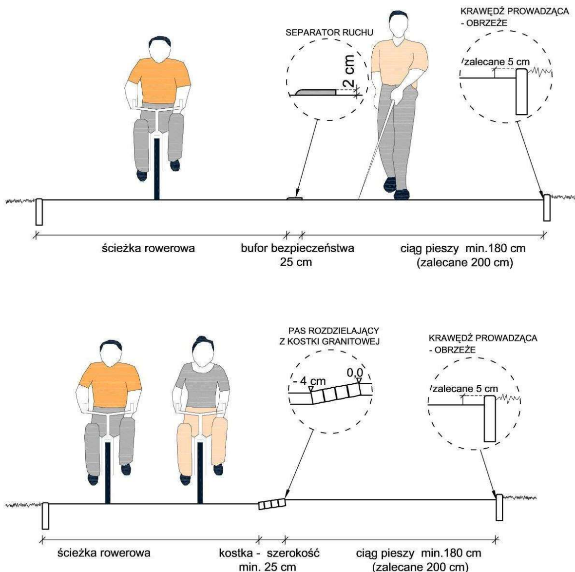
Rys. 8. Dopuszczalne rozdzielanie ścieżki rowerowej i ciągu pieszego;
