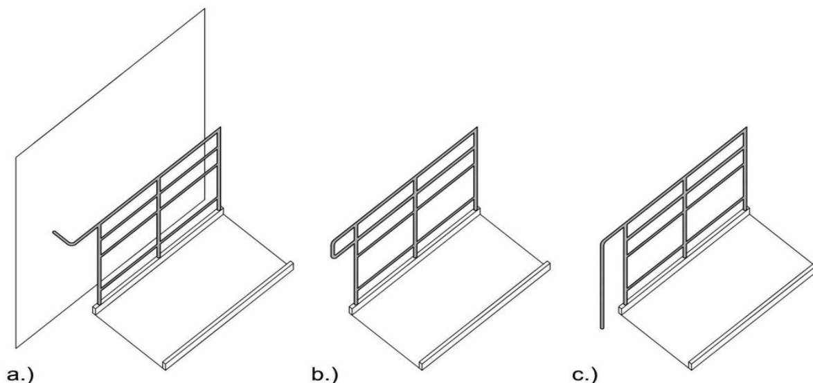
Rys. 31. Zalecane zakończenia balustrad
