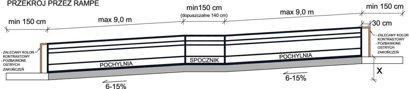
Rys. 30. Rampa dla niepełnosprawnych
