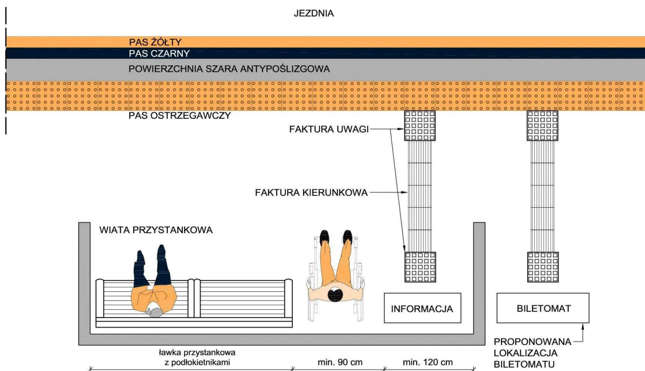
Rys. 27. Przykładowe rozplanowanie strefy niebezpiecznej i otoczenia wiaty przystankowej .
