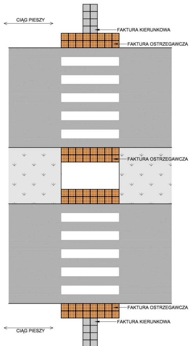
Rys. 22 Przykład zastosowania elementów systemu FON na przejściach dla pieszych z pasem dzielącym.
