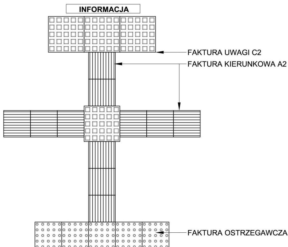
Rys. 18. Przykład zastosowania elementów systemu FON;
