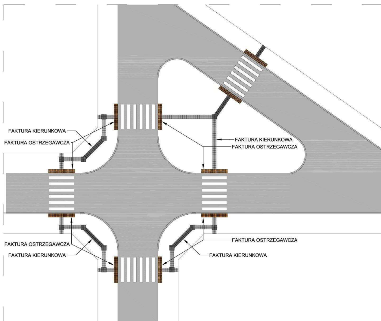
Rys. 23. Przykład zastosowania elementów systemu FON na skrzyżowaniu
