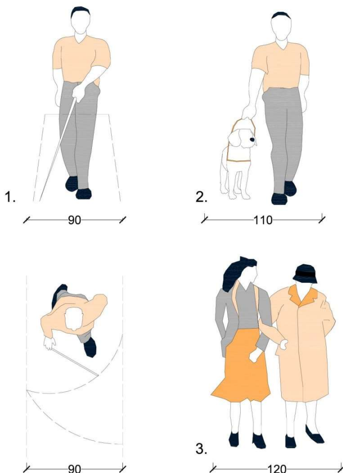
Rys. 2. [15] Minimalne wymiary skrajni potrzebne do poruszania się osób z dysfunkcjami wzroku:
