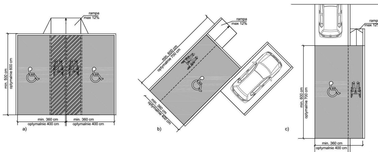
Rys. 34. Wymiary stanowisk postojowych usytuowanych przy jezdni z miejscowym obniżeniem nawierzchni chodnika do wysokości nawierzchni stanowiska postojowego – pochylnia do poziomu koperty
