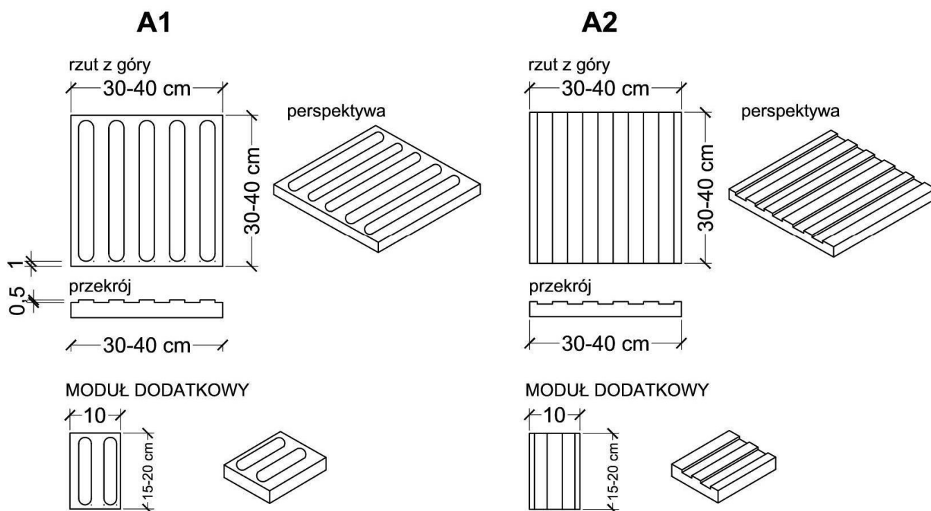
Rys. 14. [23] Płytki kierunkowe do zastosowań: A1 – na zewnątrz i wewnątrz obiektów, A3 – do wnętrza i zadaszonych peronów zewnętrznych.
