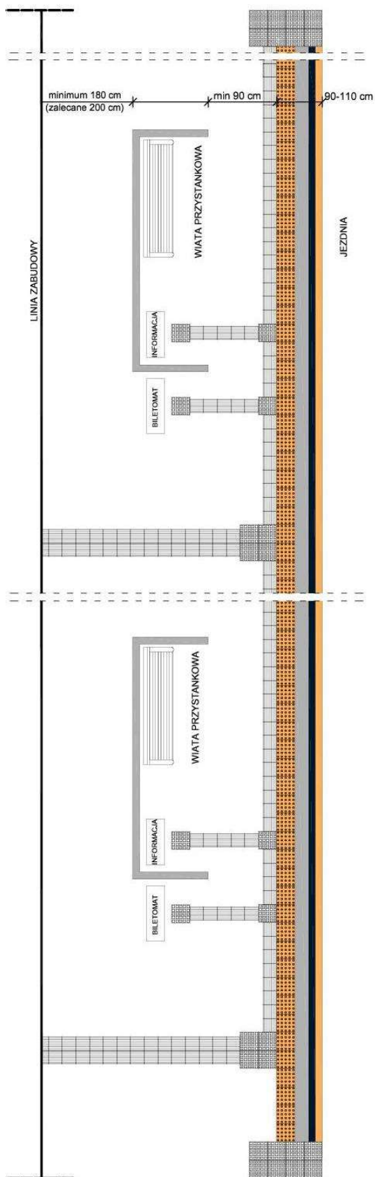
Rys. 28. Przykładowe rozplanowanie oznaczeń fakturowych na przystankach komunikacji .
