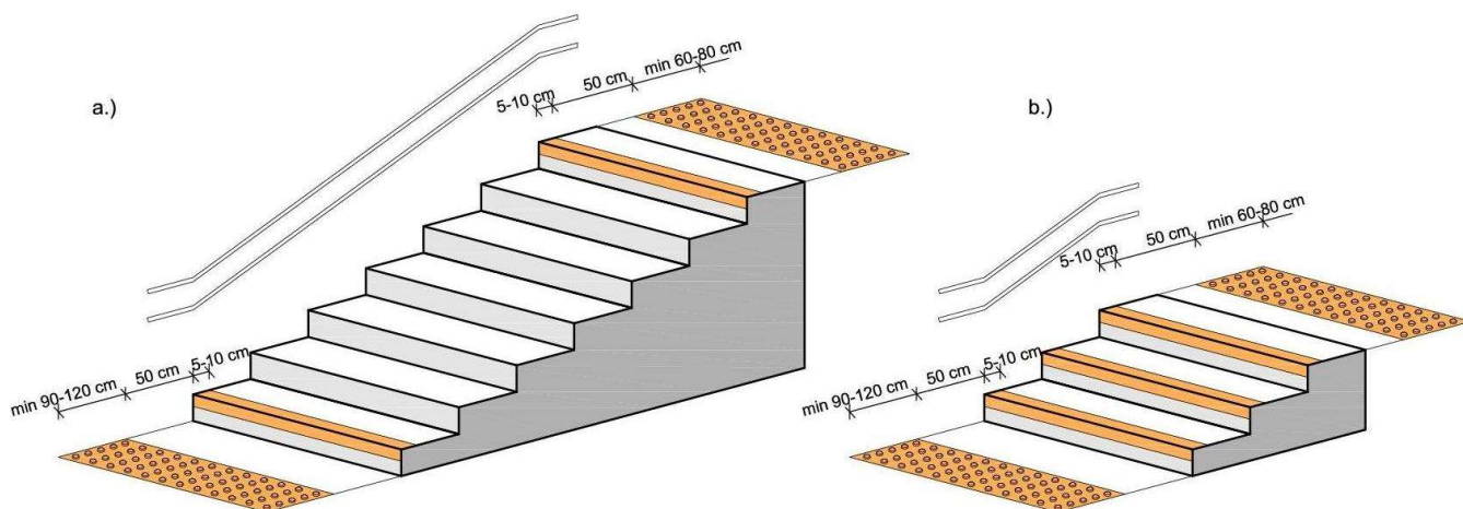
Rys. 29. Prawidłowe oznakowanie schodów:
