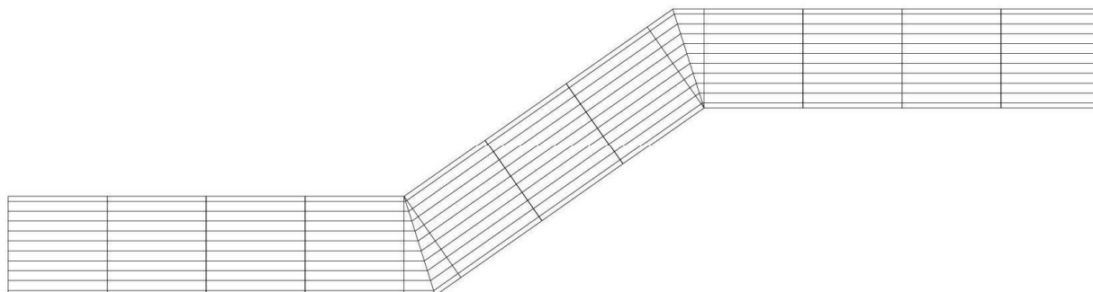
Rys. 20. Zmiana kierunku ścieżki o mniej niż 45 stopni;
