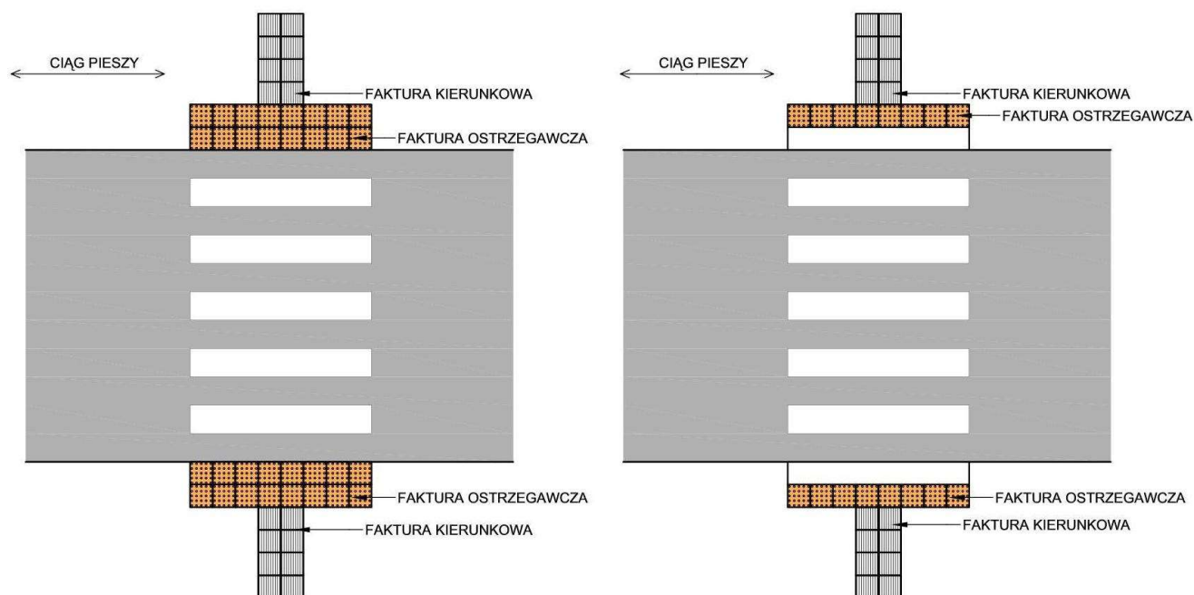
Rys. 21. Przykład zastosowania elementów systemu FON na przejściach dla pieszych.
