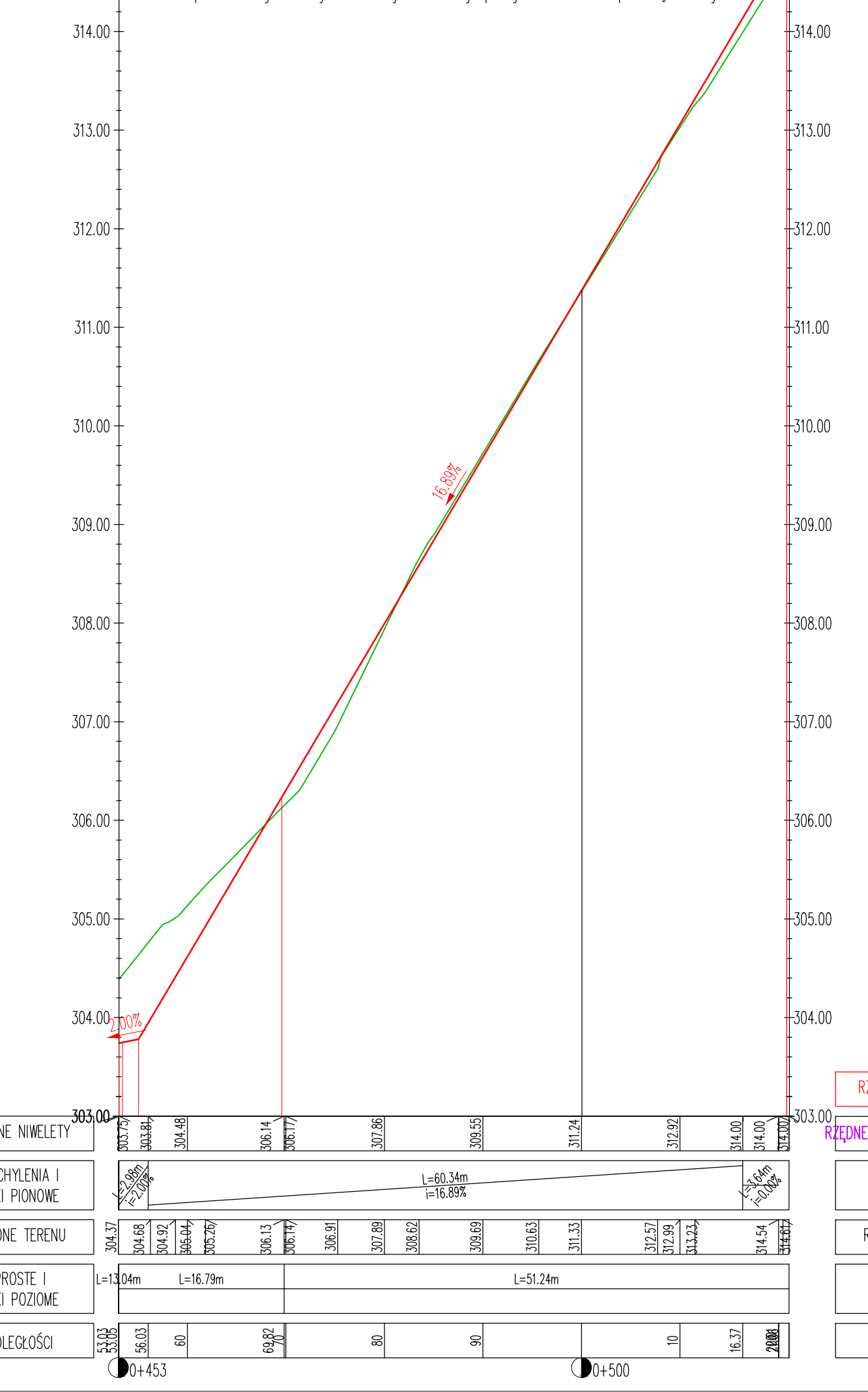
Profil podłużny - zjazd indywidualny przy numerze porządkowym 35
