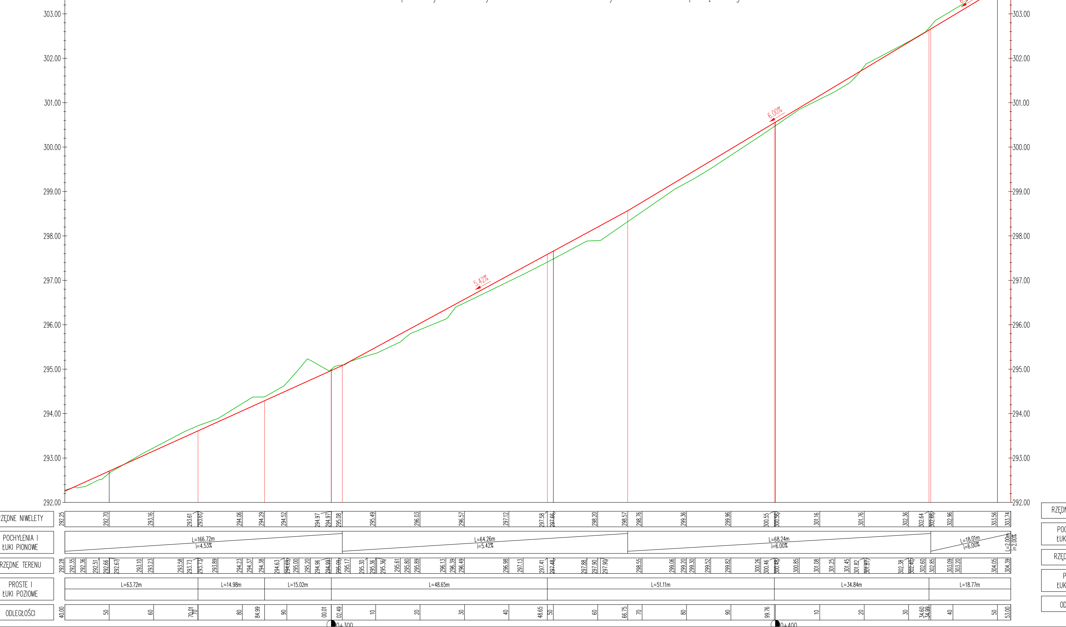
Profil podłużny ul. Świerczyńska na kierunku ul. Uniwersytecka do numeru porządkowego 35
